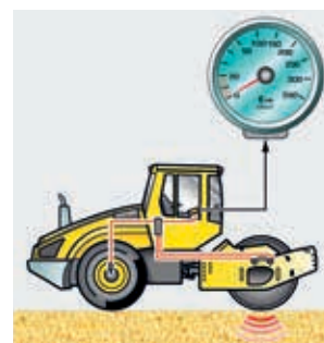
Начало: Измеритель E_{VIB} ВЕМ фирмы BOMAG.
